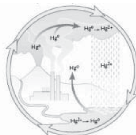
Figur 2.1 Model for kviksølvs kredsløb
